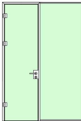
Type 680 - 35 left
